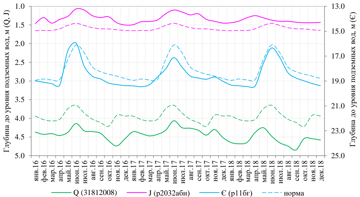
Рис. 1.25 Графики уровней подземных вод в пределах Ангаро-Ленского АБ (Сибирский САБ) в 2016–2017 гг. и прогноз на 2018 г.
