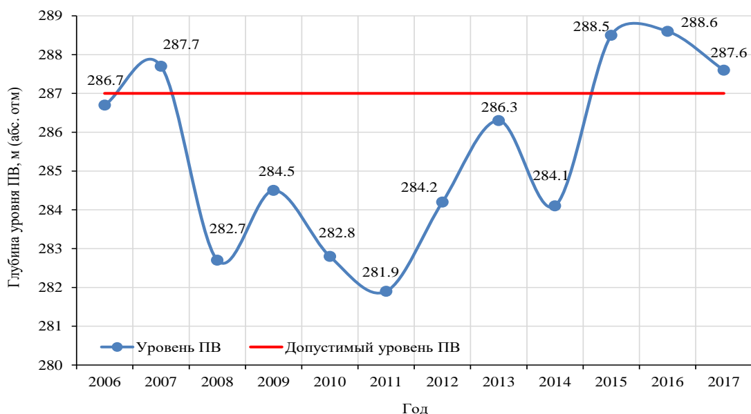
Рис. 1.38 Изменение уровней подземных вод на Майминском водозаборе в 2006-2017 гг.
