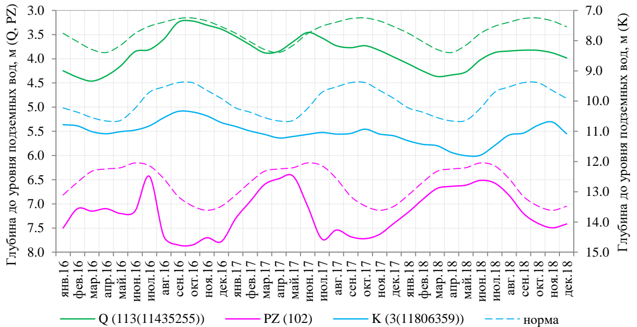
Рис. 1.26 Графики уровней подземных вод в пределах Хамардабан-Баргузинской (Q, K) и Малхано-Становой ГСО (PZ) (Байкало-Витимская СГСО) в 2016-2017 гг. и прогноз на 2018 г.
