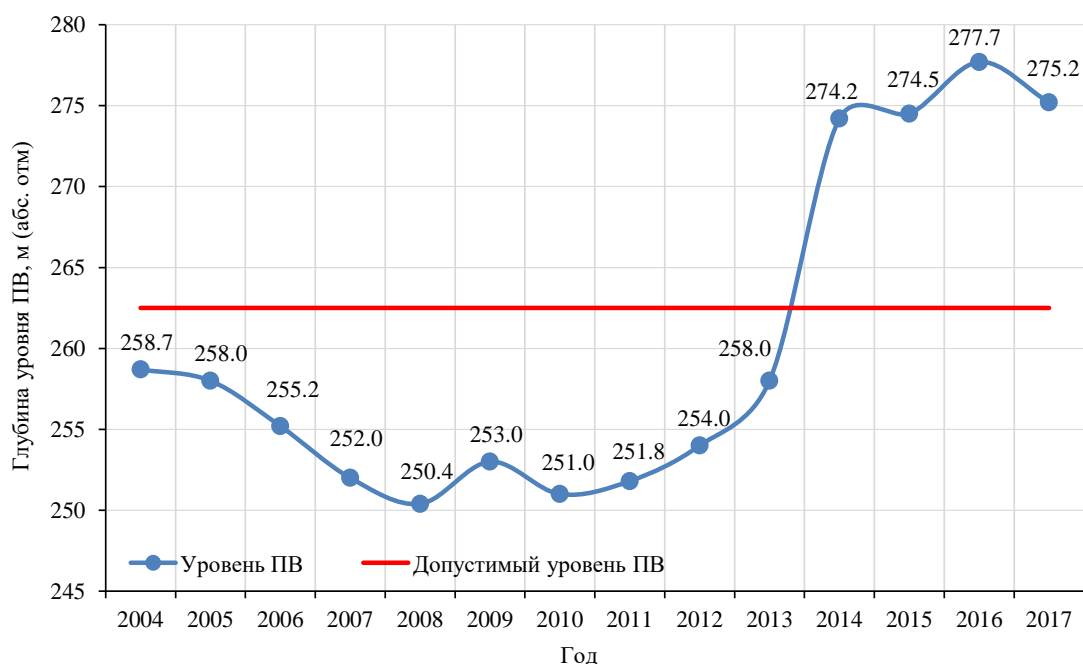
Рис. 1.39 Изменение уровней подземных вод на Улалинском водозаборе в 2004-2017 гг.
