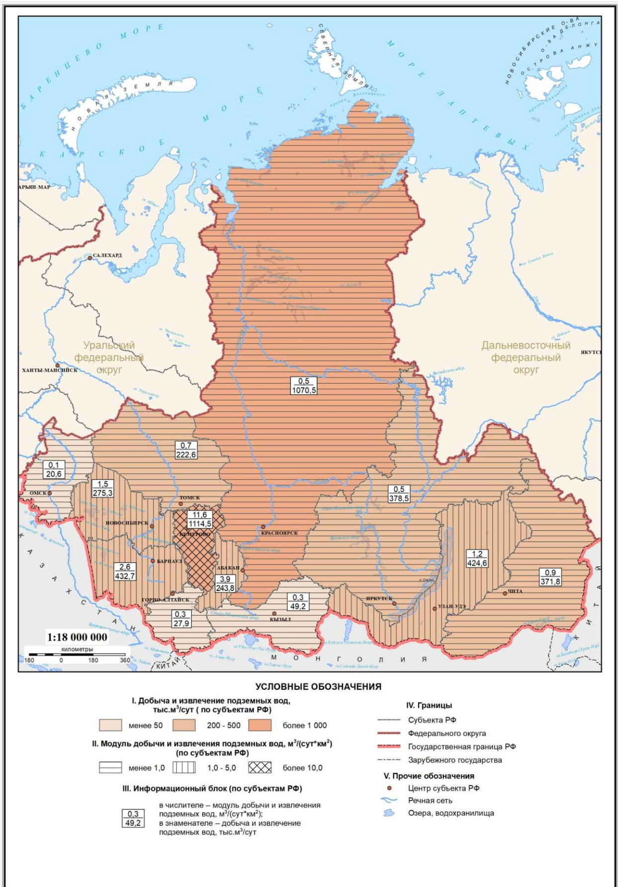
Рис. 1.23 Карта добычи и извлечения подземных вод на территории Сибирского федерального округа в 2017 году. Масштаб 1:18 000 000
