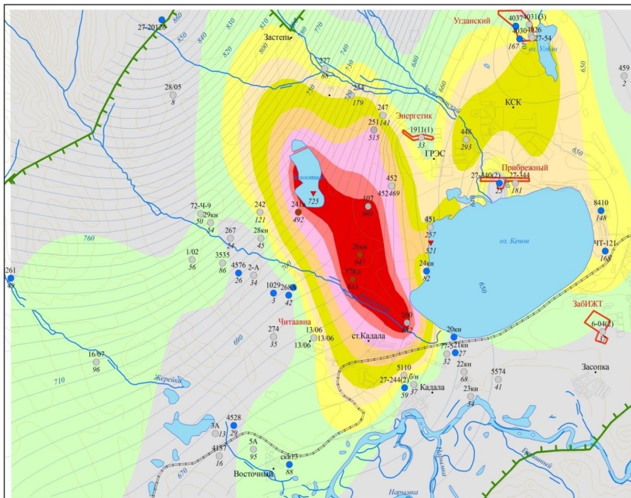
Масштаб 1:75 000 0 1,25 2,5 5 7,5 10км Рис. 1.41 Распространение сульфатов в подземных водах в районе гидрозолоотвала ТЭС-1 в 2017 г.
