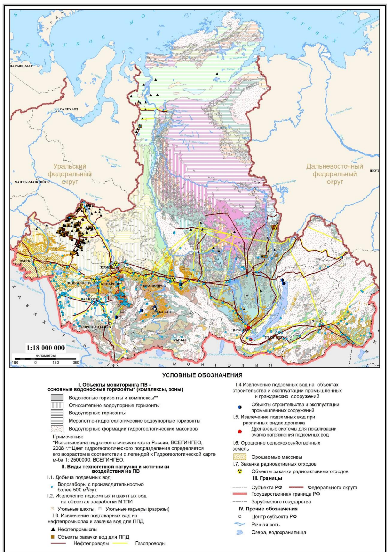
Рис. 1.3 Карта техногенной нагрузки на территории СФО. Масштаб 1:18 000 000
