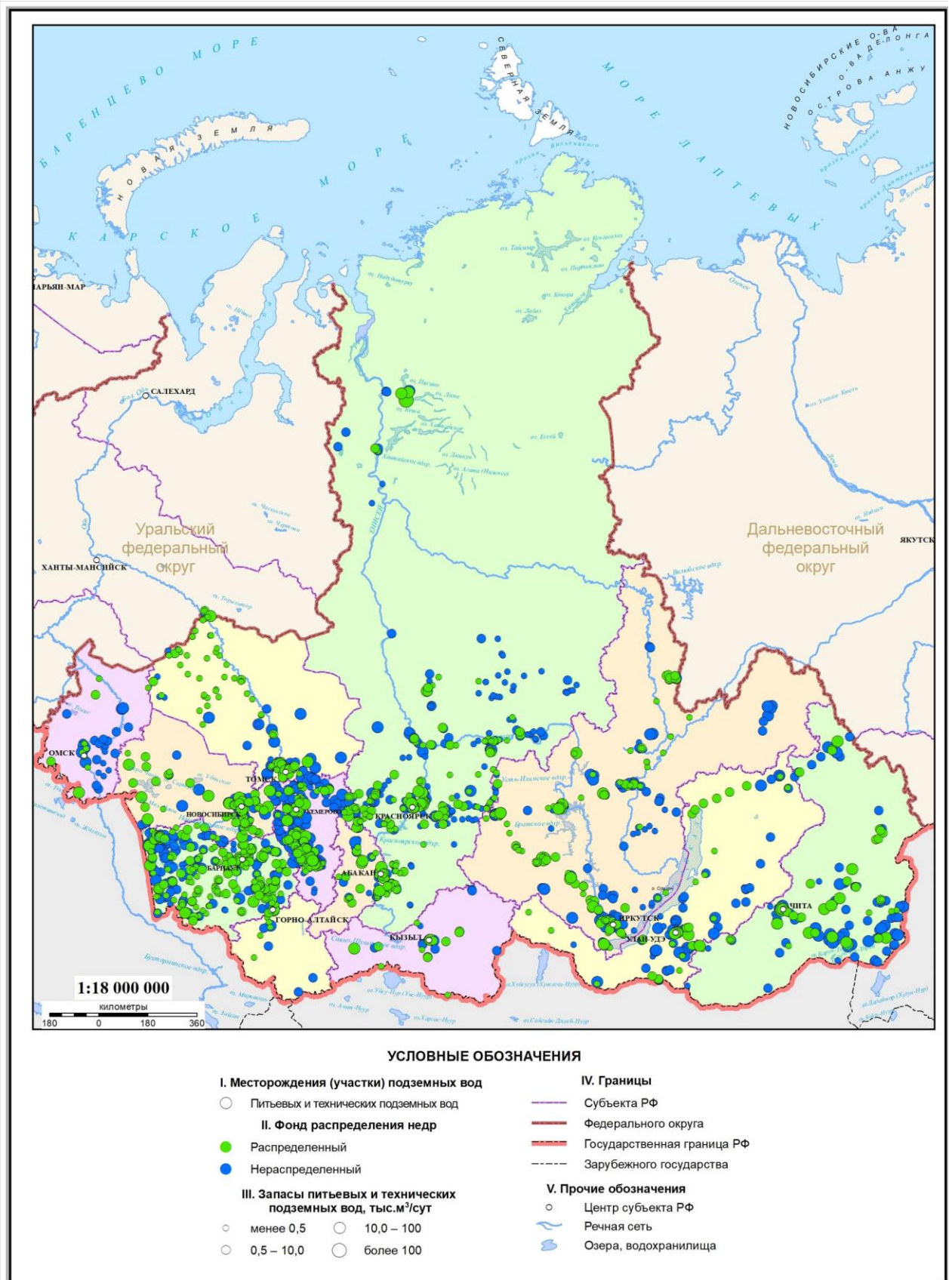
Рис. 1.12 Карта месторождений пресных подземных вод на территории СФО (по состоянию на 01.01.2018 г.). Масштаб 1:18 000 000
