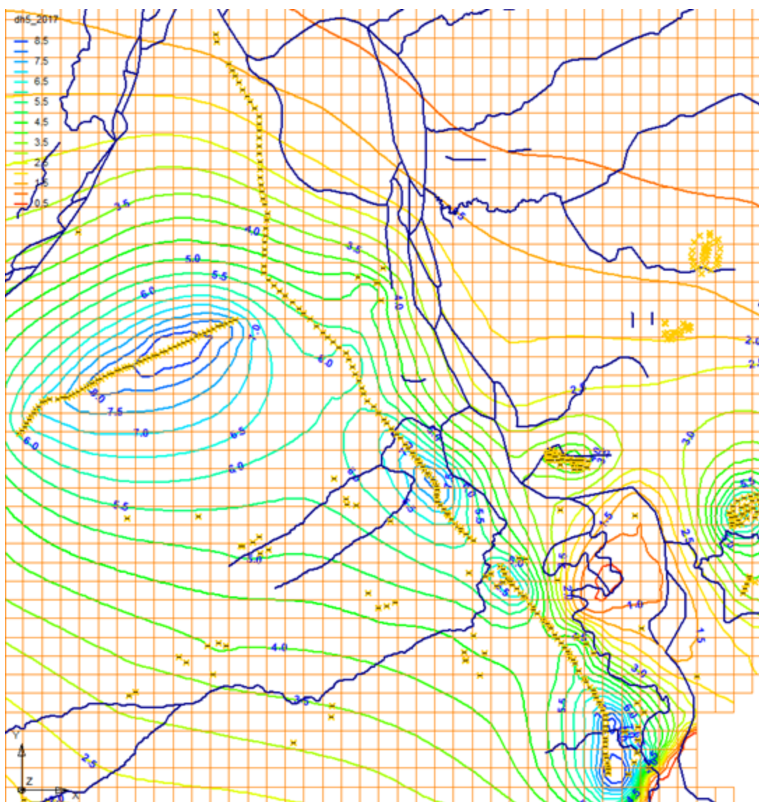
Рис. 1.43 Понижение уровня подземных вод (м) в палеогеновом комплексе с начала эксплуатации водозабора
