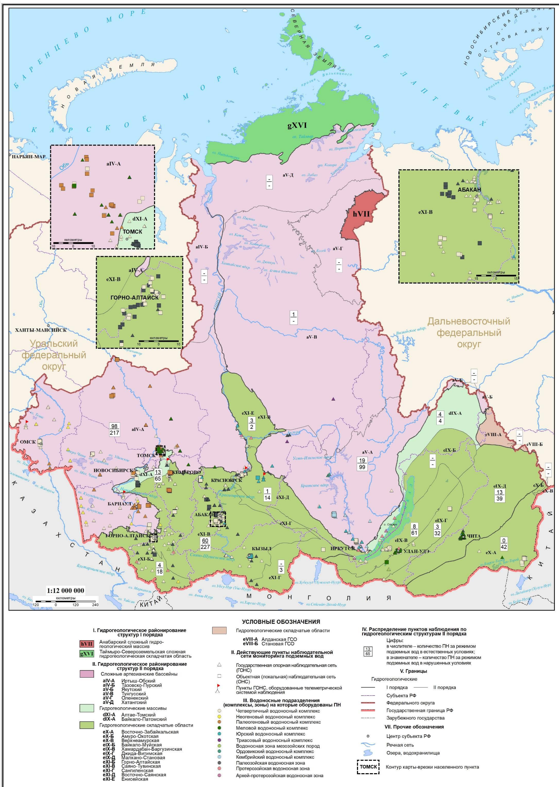
Рис. 1.5 Карта наблюдательной сети мониторинга подземных вод на территории СФО (по состоянию на 01.01.2018 г.). Масштаб 1:12 000 000
