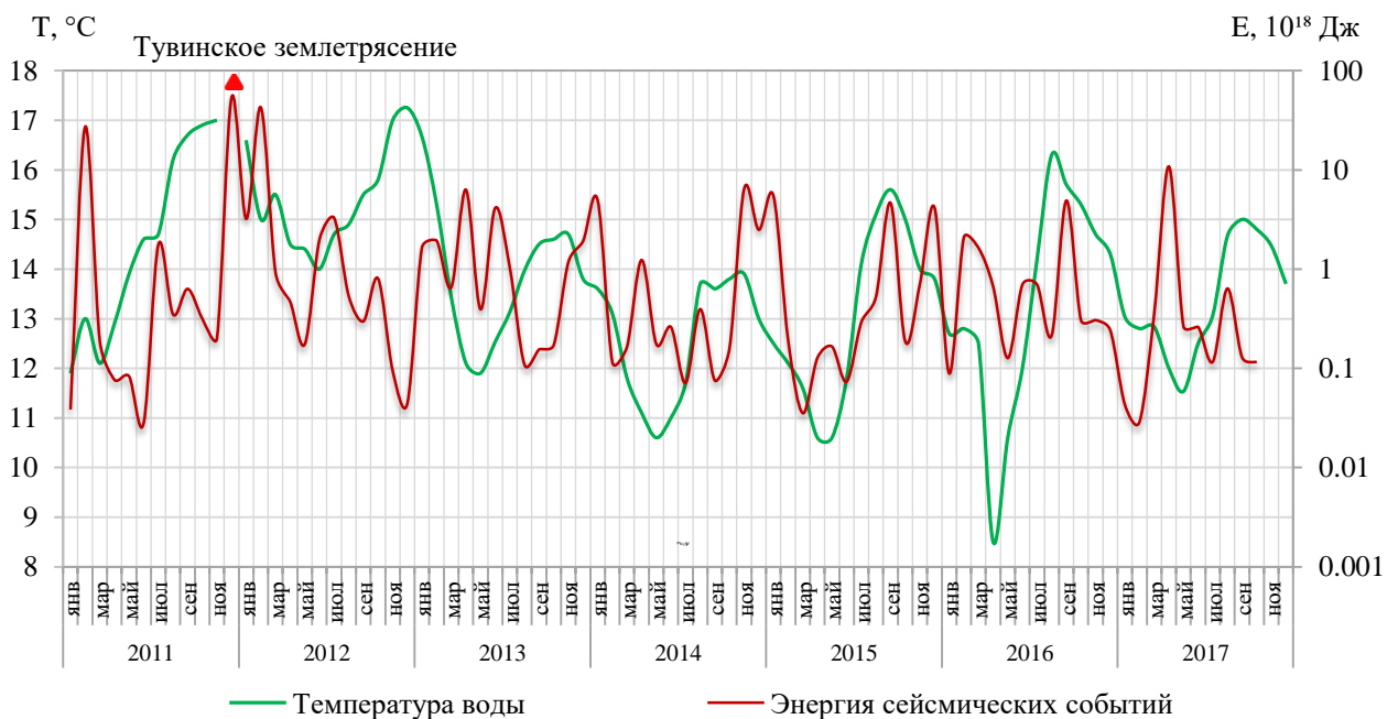
Рис. 1.28 Сопоставление температурного режима подземных вод в колонке НП «Северный» г. Горно-Алтайска и энергии сейсмических событий
