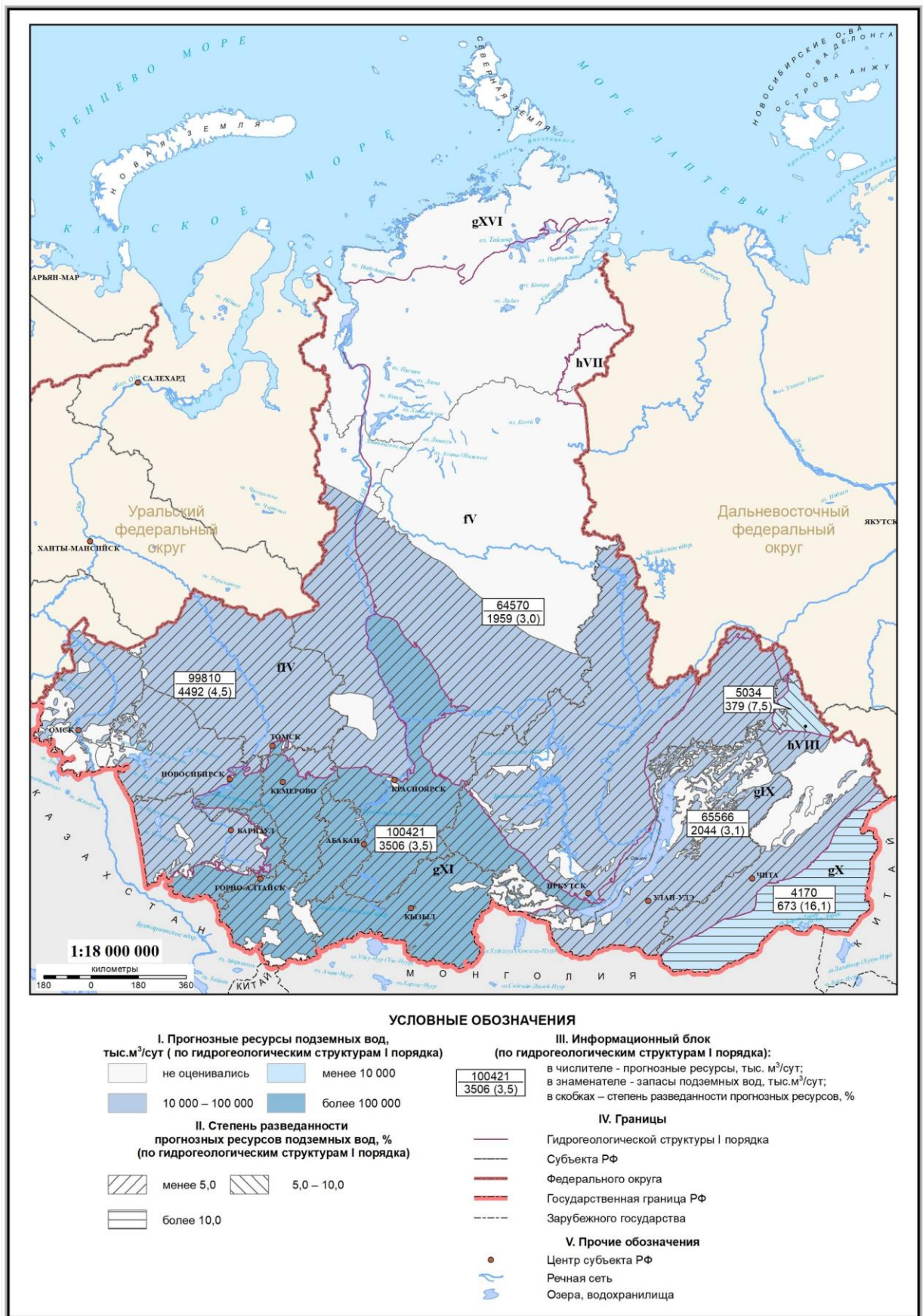
Рис. 1.9 Карта прогнозных ресурсов подземных вод и степени их разведанности по гидрогеологическим структурам I порядка на территории СФО (по состоянию на 01.01.2018 г.). Масштаб 1:18 000 000
