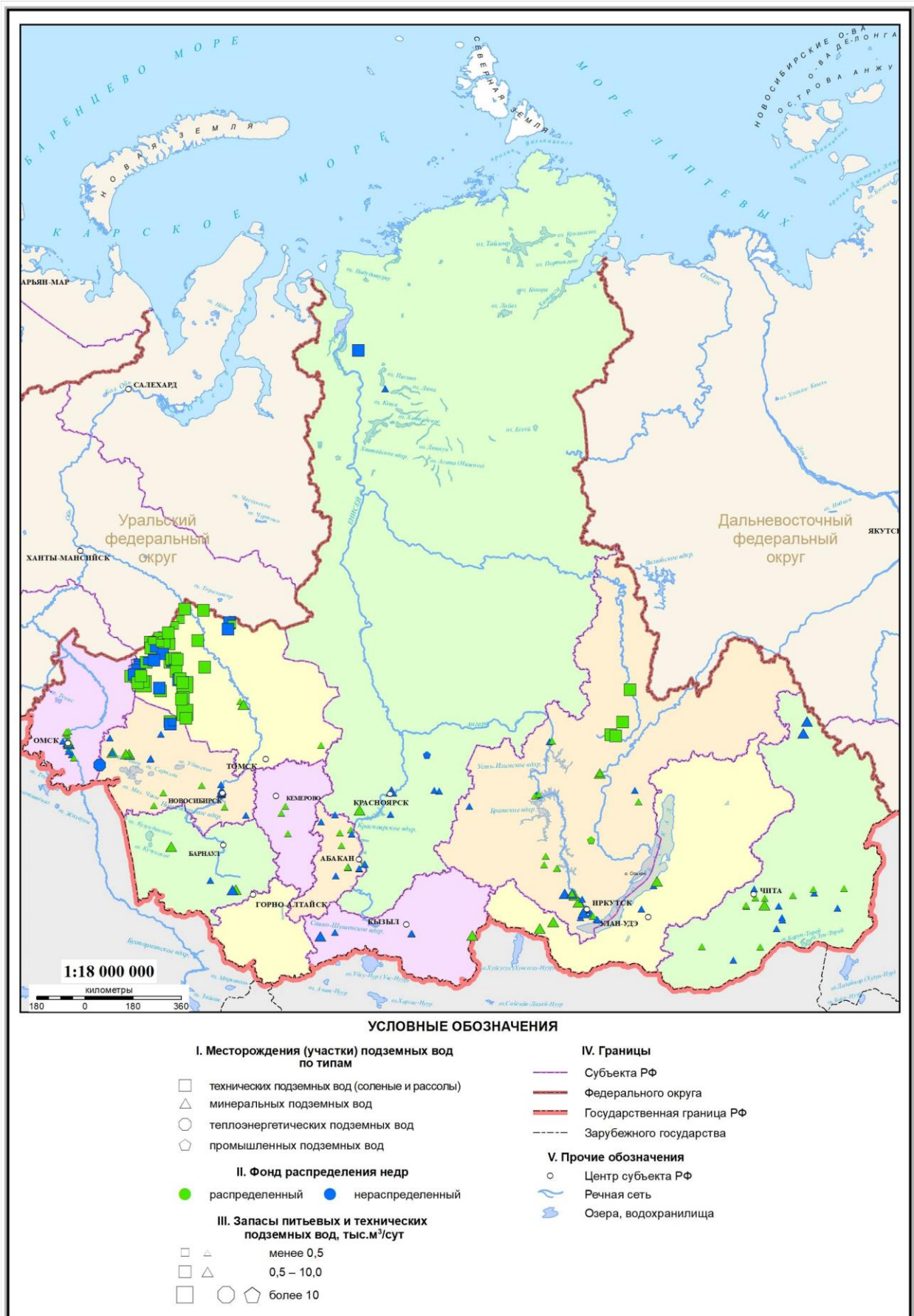
Рис. 1.18 Карта месторождений технических (соленые и рассолы), минеральных, теплоэнергетических и промышленных подземных вод на территории СФО (по состоянию на 01.01.2018 г.). Масштаб 1:18 000 000
