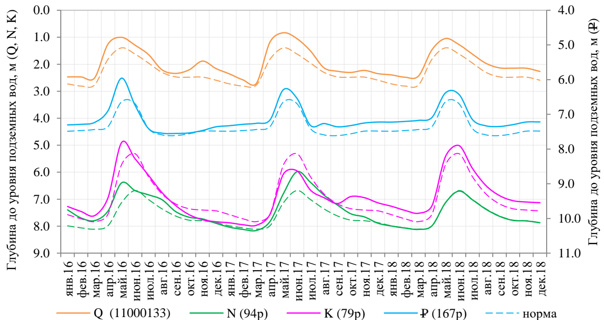
Рис. 1.24 Графики уровней подземных вод в пределах Иртыш-Обского АБ (Западно-Сибирский САБ) в 2016-2017 гг. и прогноз на 2018 г.
