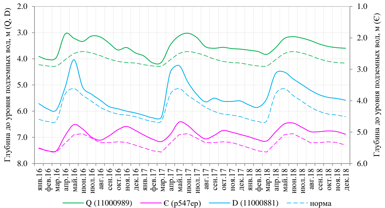
Рис. 1.27 Графики уровней подземных вод в пределах Алтае-Томского ГМ (Q, D) и Саяно-Тувинской ГСО (€) (Алтае-Саянская СГСО) в 2016–2017 гг. и прогноз на 2018 г.
