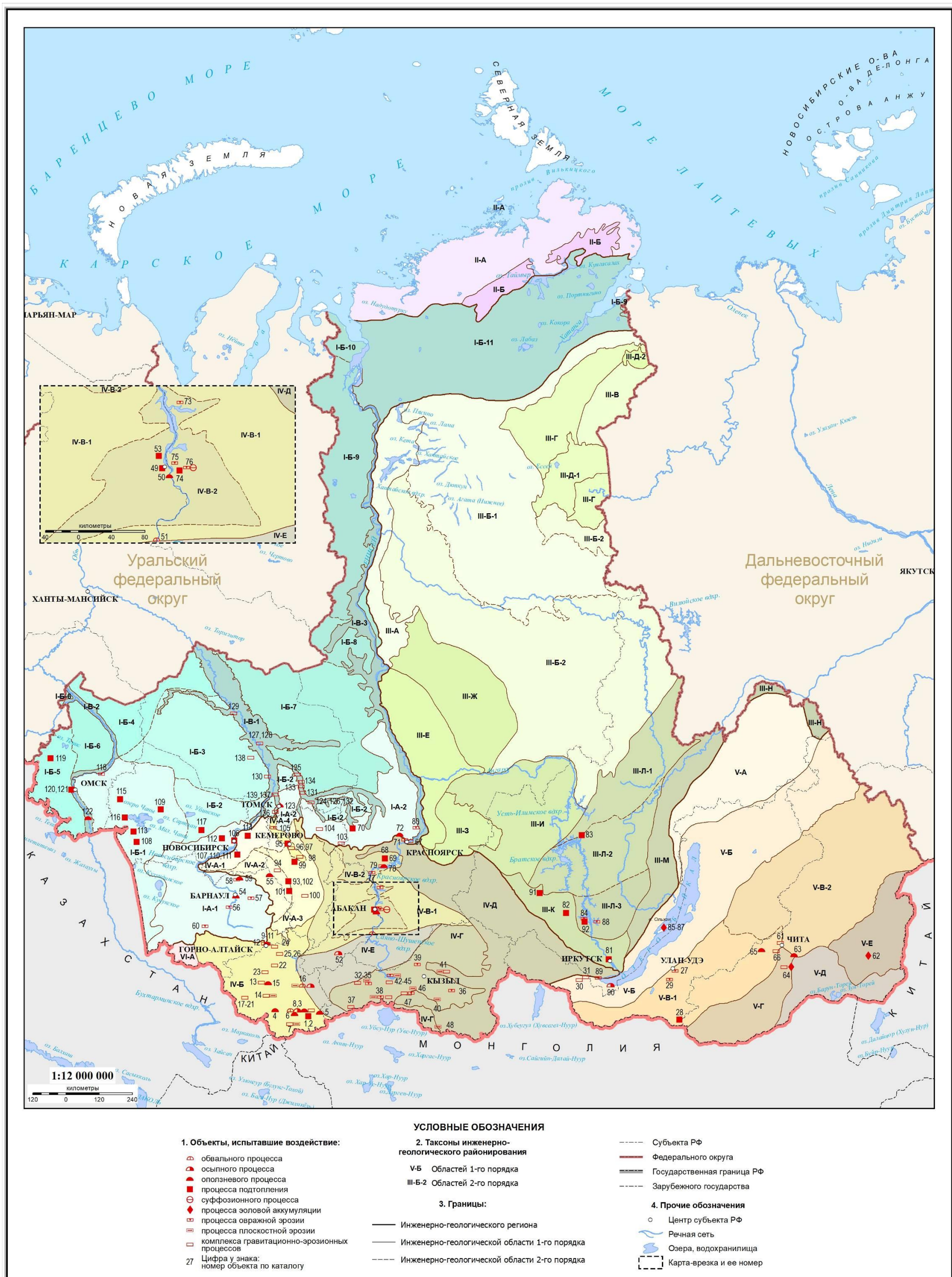
Рис. 2.31 Карта объектов, испытавших воздействие опасных ЭГП на территории СФО (по состоянию на 01.01.2018 г.). Масштаб 1:12 000 000
