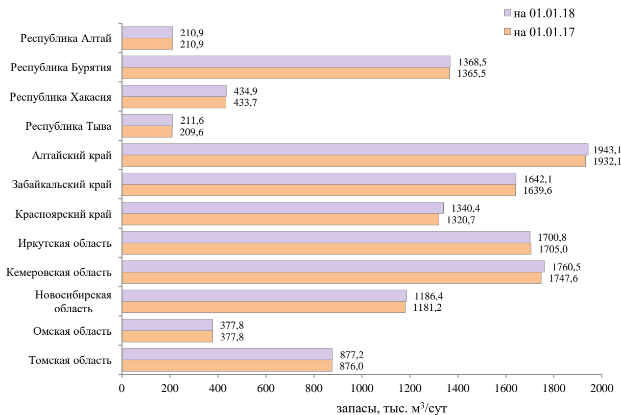
Рис. 1.13 Изменение балансовых запасов питьевых и технических (пресных и слабосоленых) подземных вод по субъектам РФ на территории СФО
