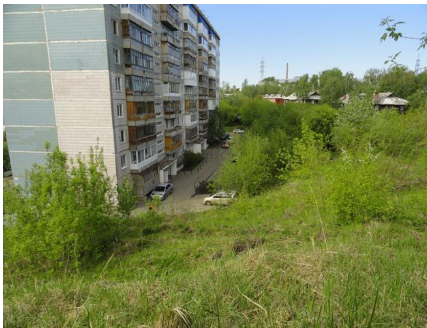
Рис. 2.21 Оползневой склон в мкр. Солнечный в г. Томске, Томская область
