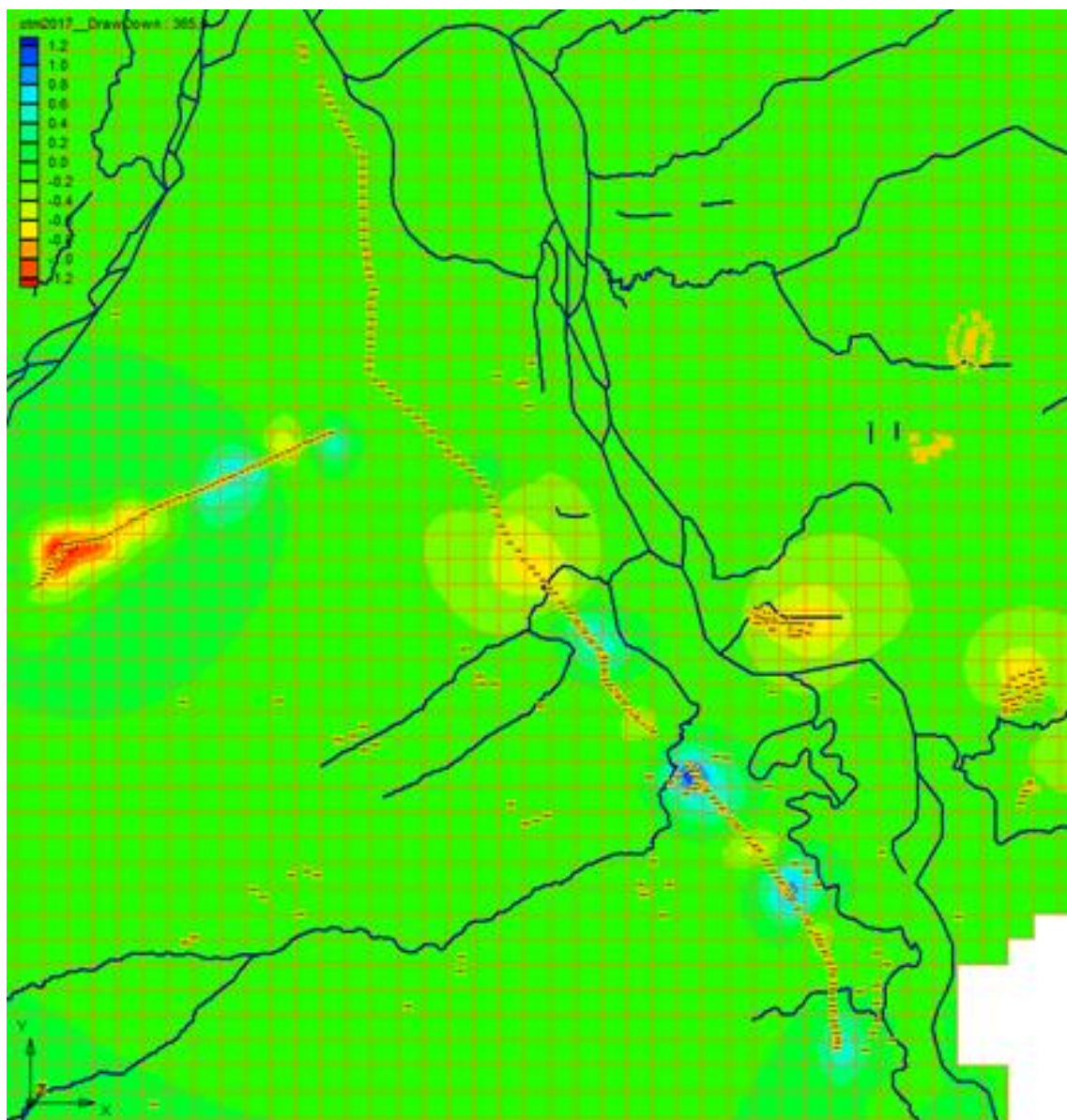
Рис. 1.42 Изменение уровня подземных вод в палеогеновом комплексе, м (по состоянию на 01.01.2018 г.)
