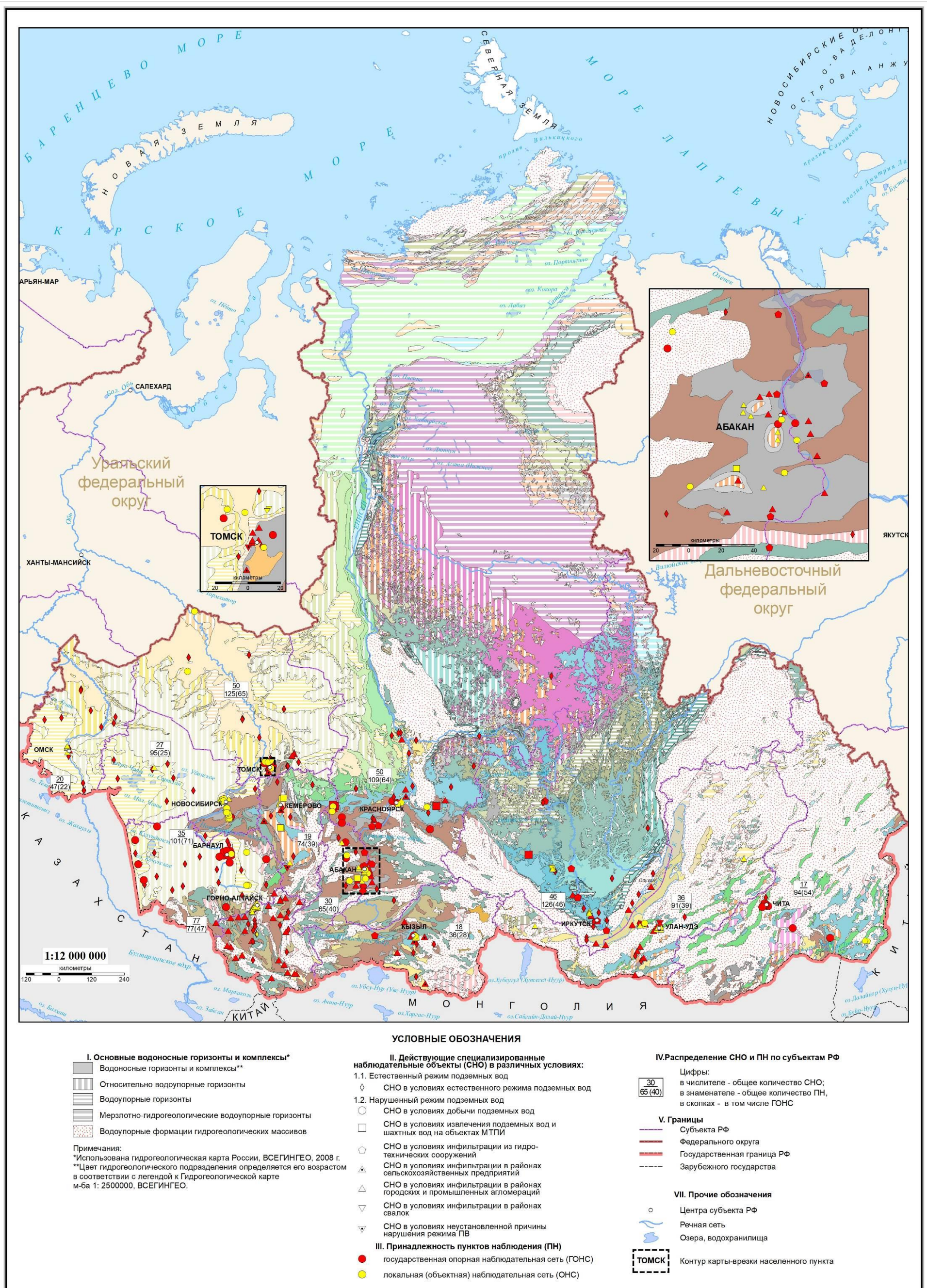
Рис. 1.4 Карта СНО в различных условиях режима подземных вод на территории СФО (по состоянию на 01.01.2018 г.). Масштаб 1:12 000 000
