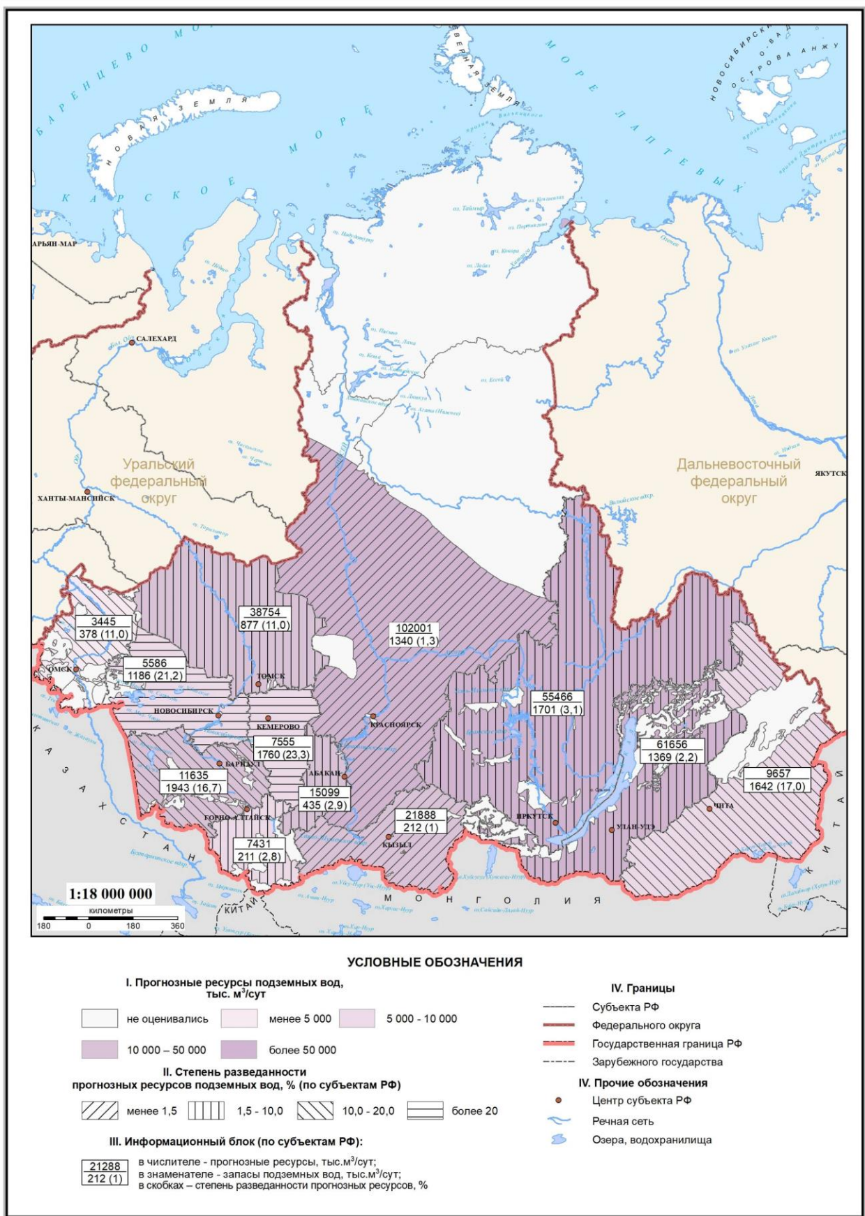
Рис. 1.8 Карта прогнозных ресурсов подземных вод и степени их разведанности по субъектам РФ на территории СФО (по состоянию на 01.01.2018 г.). Масштаб 1:18 000 000
