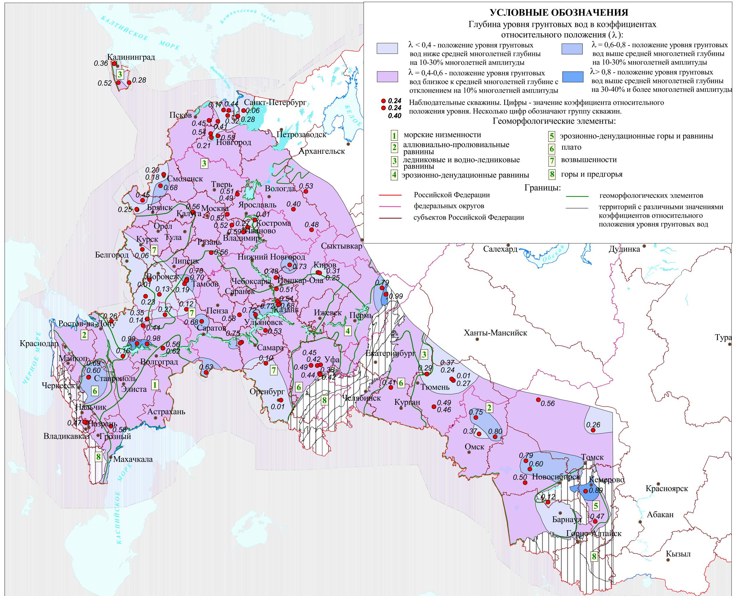
Рис. 1. Карта прогнозных весенних максимальных уровней грунтовых вод Европейской части России и юга Западной Сибири на 2015 год (уточненный прогноз)
