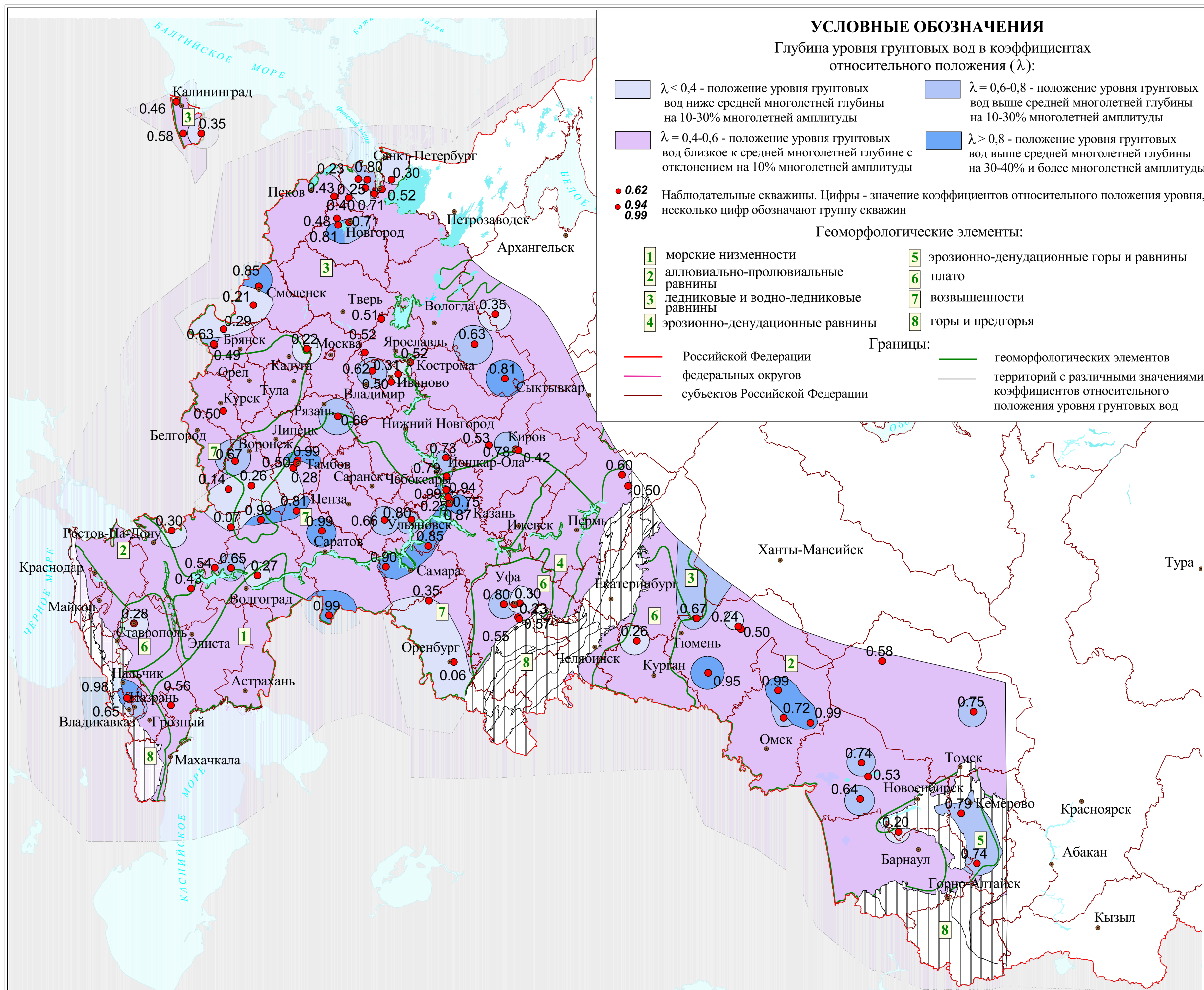
Рис. 1. Карта прогнозных осенне-зимних минимальных уровней грунтовых вод Европейской территории России и юга Западной Сибири на 2018 год (уточненный прогноз)
