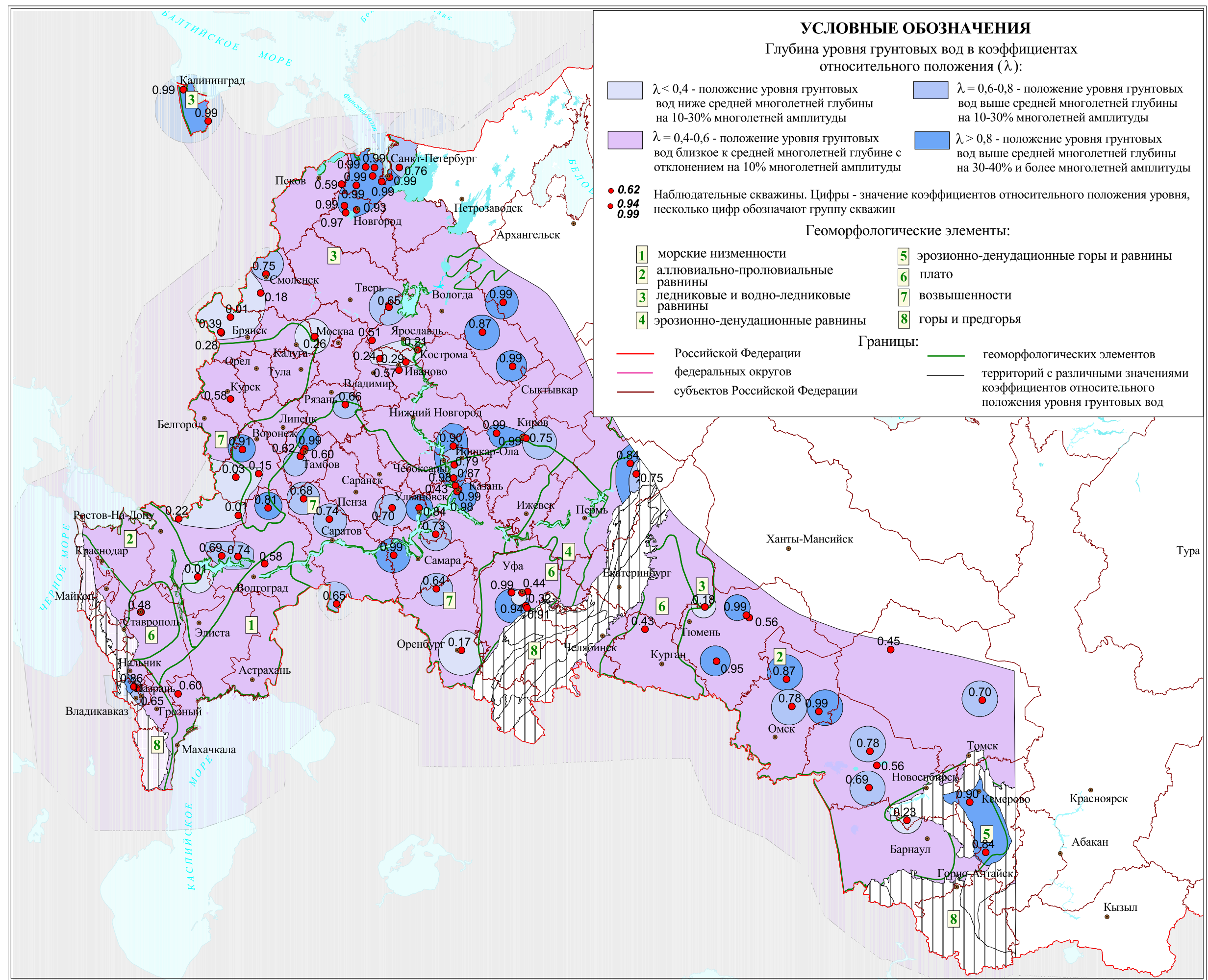
Рис.2. Карта фактических осенне-зимних минимальных уровней грунтовых вод Европейской территории России и юга Западной Сибири в 2017 году
